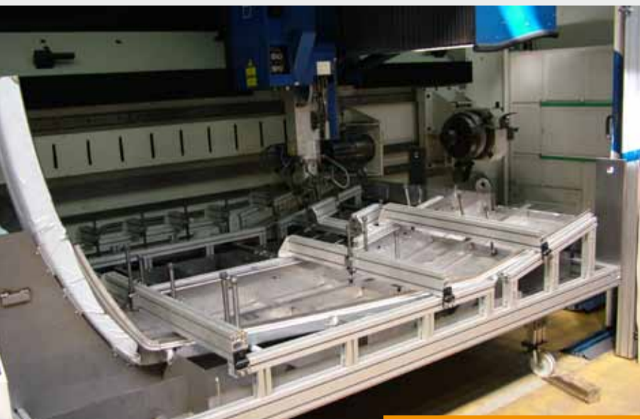
Laserschweißvorrichtung DT5-Kopf Hamburger Hochbahn
